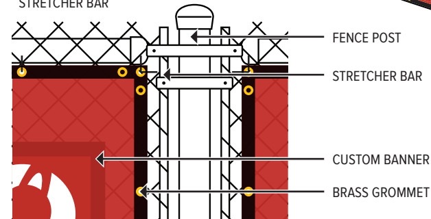
STRETCHER BAR
